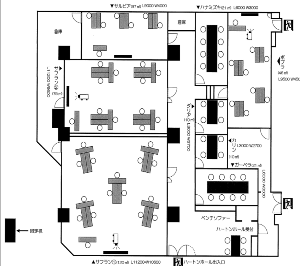
ハートンホール毎日新聞ビルB1 全体平面図 1/150
